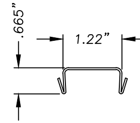
23 DOOR TOP RAIL .06" THK. STEEL
