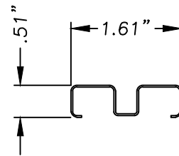
13 DOOR BOTTOM RAIL .06" THK. STEEL
