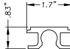
(29)(30) FLUSH BOLT TOP / BOTTOM ALUMINUM 6063-T5
